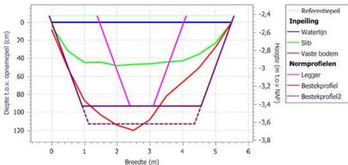
Figuur 6: illustratie normprofielen waterlichaam
